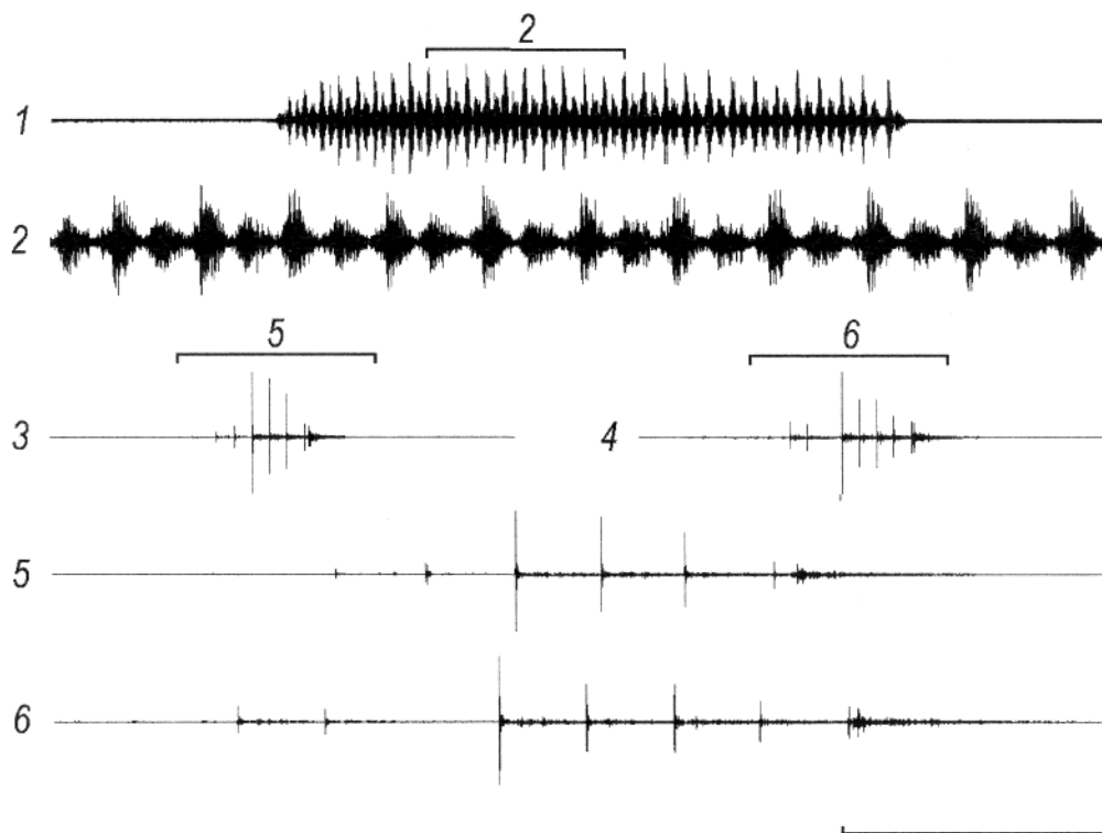
Рис. 2. Осциллограммы звуковых сигналов самцов Acrida bicolor (Thnb.), издаваемых тегмино-фemorальным акустическим аппаратом (1-2) и в полете (3-6) при разной временной развертке. 1-2 — одиночный самец с одной правой задней ногой; 3-6 — в полете после вспугивания. Отметка времени внизу для осциллограмм 1, 3, 4 — 500 мс; 2, 5, 6 — 100 мс
